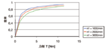
力矩作用下的行星齿轮箱的效率曲线示例
