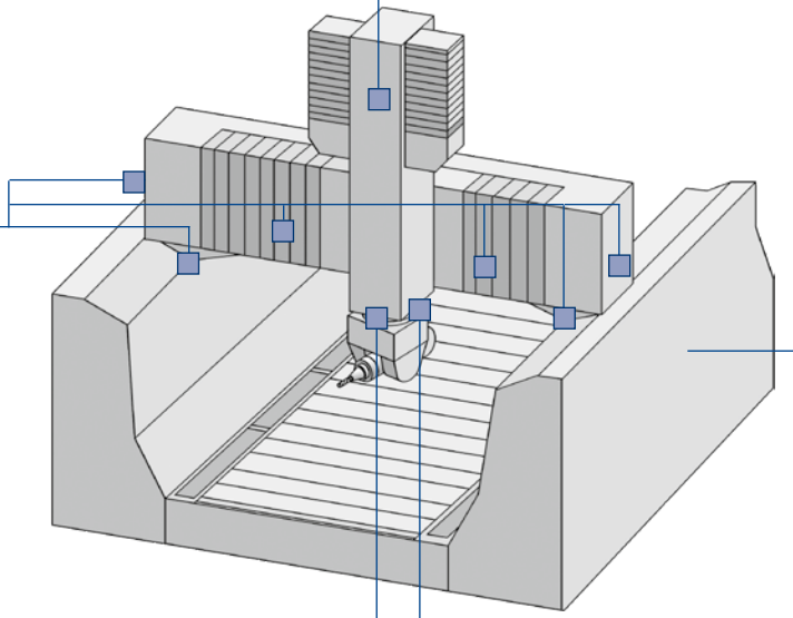
适用于所有轴的 润滑系统
